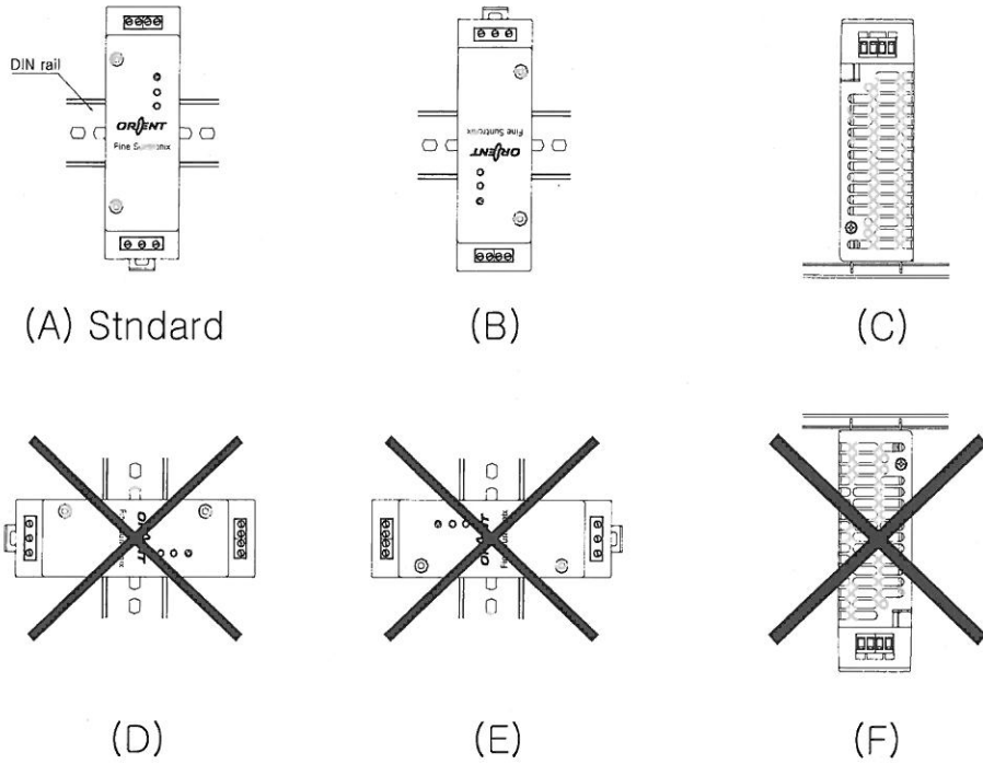
< Fig.10 제품 실장 예 >
