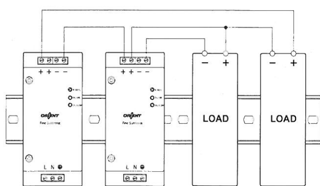
< Fig.3 직렬운전 B >
