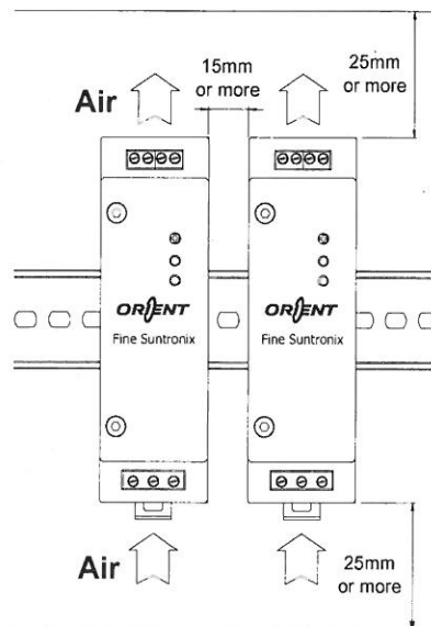
< Fig.9 실장 방법 >
