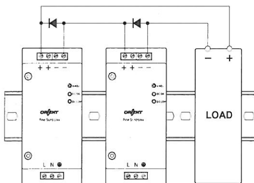
< Fig.2 직렬운전 A >
