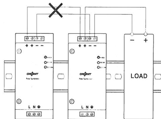
< Fig.5 병렬운전 B (사용불가) >
