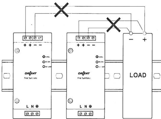
< Fig.4 병렬운전 A (사용불가) >
