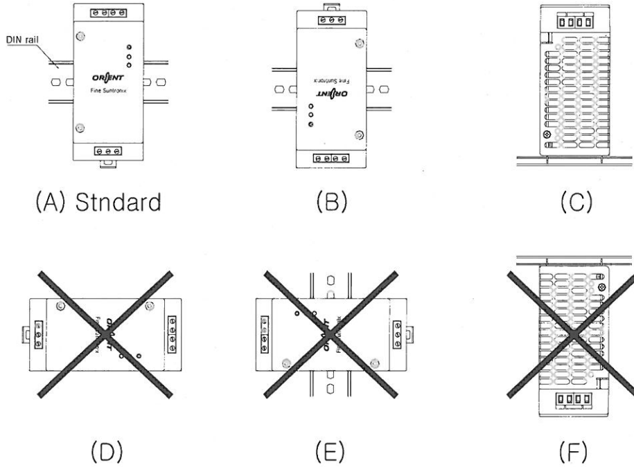
< Fig.10 제품 실장 예 >
