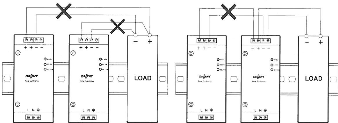
< Fig.4 병렬운전 A (사용불가) >
