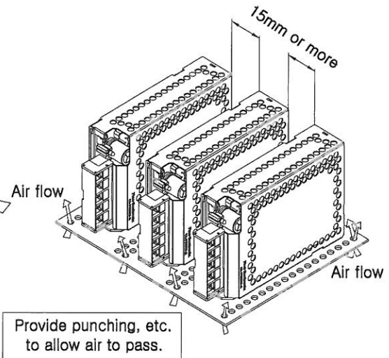
Fig 2. 응용 실장법
